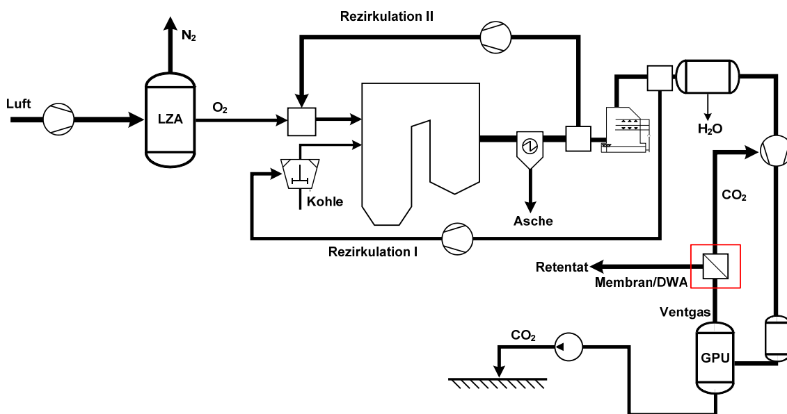
Abbildung 2: Oxyfuel-Prozess mit kryogener LZA und erhöhter CO 2 -Abtrennungsrate
