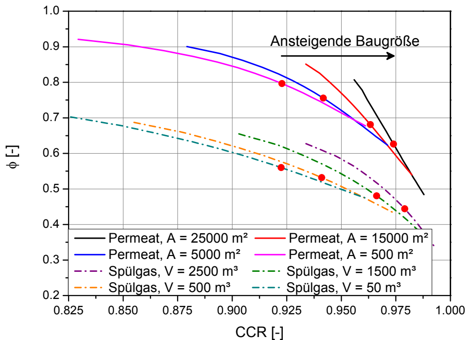
Abbildung 38: CO 2 -Konzentration \phi in Abhängigkeit von der Gesamtabtrennungsrate CCR und der Membranfläche A bzw. dem DWA-Volumen V; \Pi_{Zus} = 4 ; Punkte: Gesamtabtrennungsrate CCR, ab der eine Konzentration von \psi = 96 Vol.-% unterschritten wird
