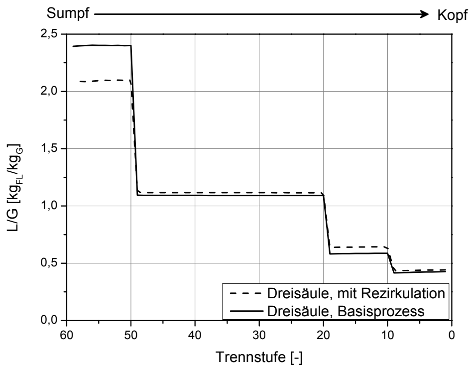
Abbildung 58: L/G-Verhältnis der ND-Kolonnenne des Dreisäulenprozesses für den Basisprozess und den Prozess mit einer Rezirkulation des Retentats
