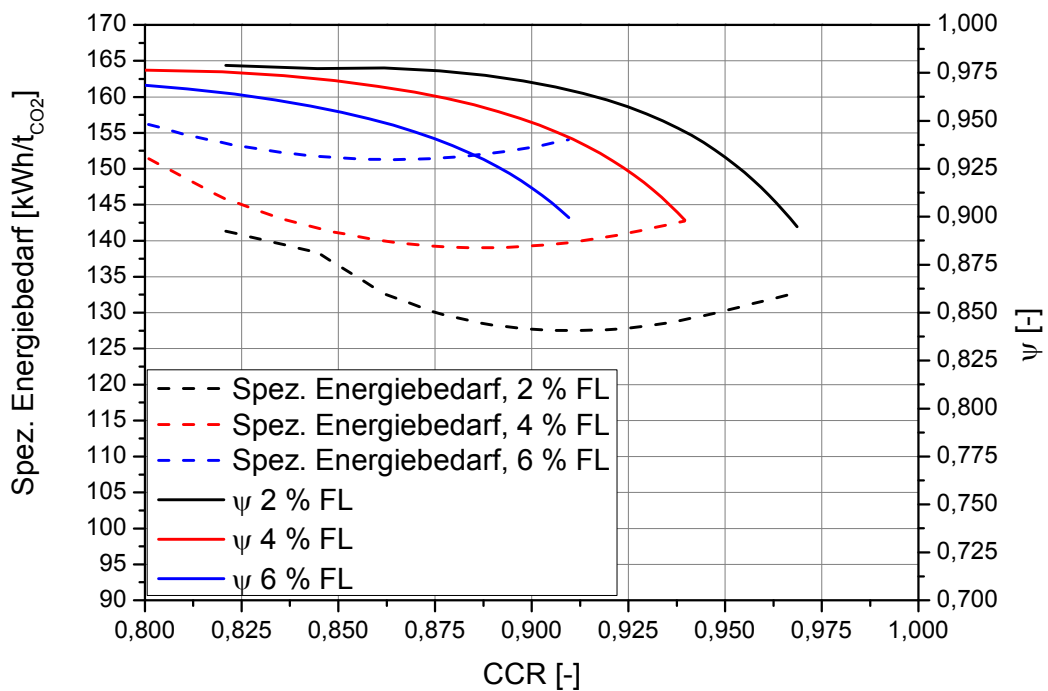
Abbildung 26: Spezifischer Energiebedarf der CO 2 -Abtrennungsanlage und CO 2 -Konzentration \psi in Abhängigkeit von der CO 2 -Abtrennungsrate CCR und vom Falschlufteintrag
