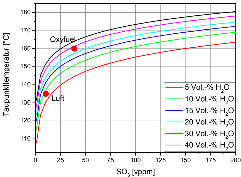
Abbildung 6: Schwefelsäuretaupunkttemperatur für Rauchgase in Abhängigkeit von den SO 3 - und H 2 O-Konzentrationen im Rauchgas nach [87]; Punkte: Ergebnisse südafrikanische Steinkohle
