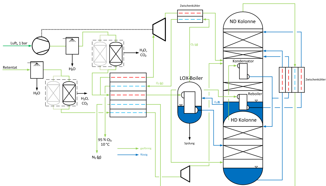
Abbildung 55: Doppelsäulenprozess mit integrierter Retentatrezirkulation; Retentat wird in der ND-Kolonne zugeführt
