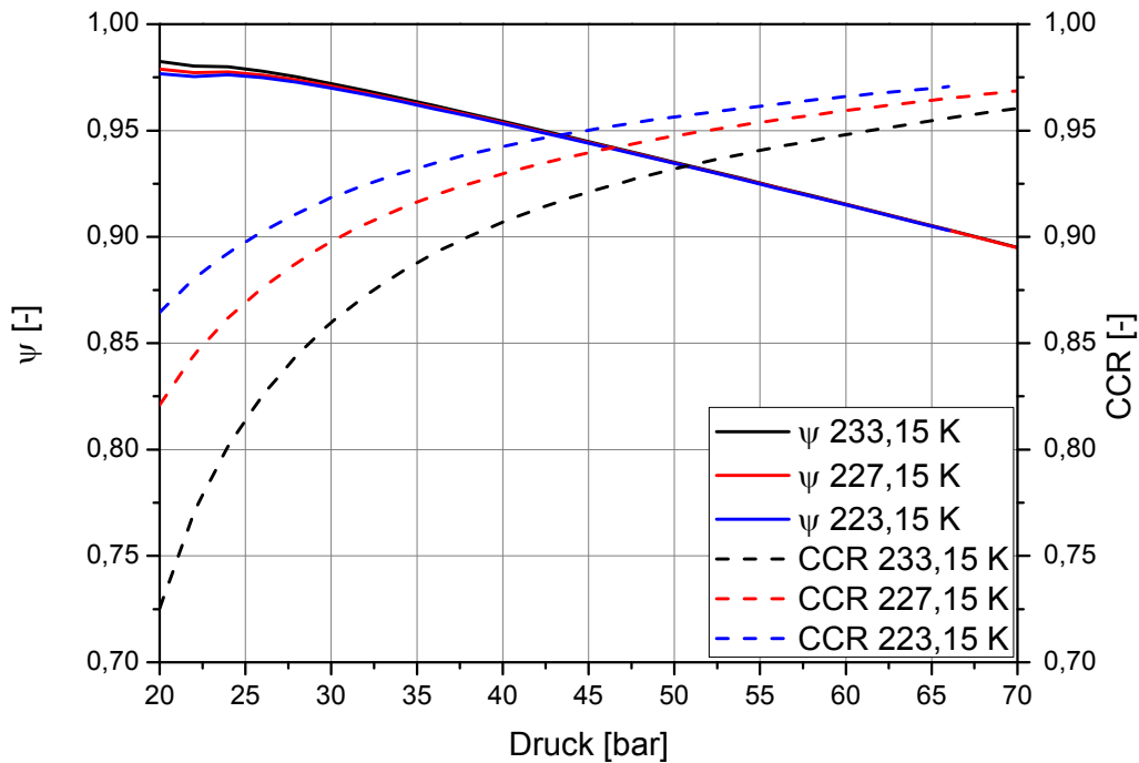
Abbildung 25: CO 2 -Konzentration \psi und CO 2 -Abtrennungsrate CCR des extern gekühlten CO 2 -Abtrennungsprozesses mit zweistufiger partieller Kondensation in Abhängigkeit vom Rauchgasverdichteraustrittsdruck und von der Temperatur des zweiten Abtrenners; Falschlufteintrag 2 %
