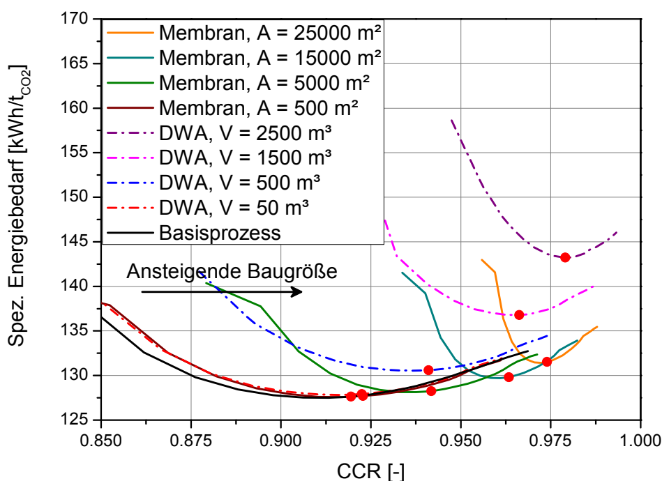
Abbildung 40: Spezifischer Energiebedarf der GPU in Abhängigkeit von der CO 2 -Abtrennungsrate CCR und der Baugröße des zusätzlichen Abtrennungsprozesses; \Pi_{\text{zus}} = 4 ; Punkte: CCR, ab dem \psi = 96 Vol.-% unterschritten wird
