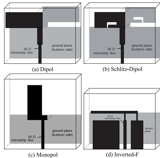
Abb. 2. Überblick verwendeter generischer PCB-Antennen.
