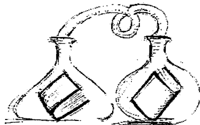
CHEMIE
