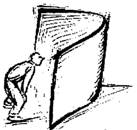
INFORMATIK
