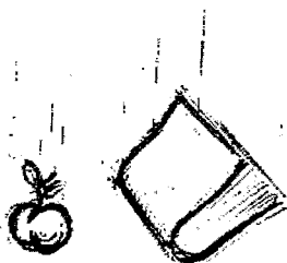
PHYSIK
