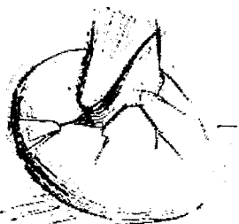
BIOLOGIE
