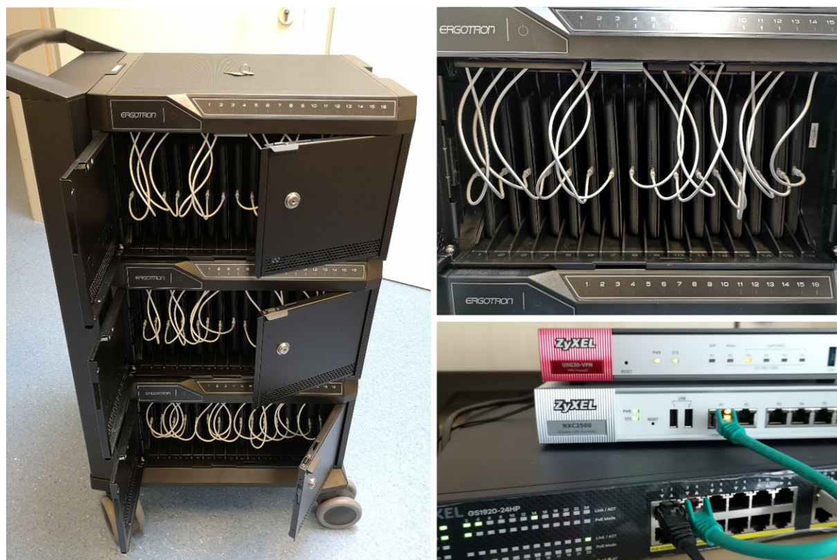
Abbildung 1: Portable Wagen (iPads) zur Lagerung und Administration der Prüfungsgeräte (links, rechts oben) sowie portabler Switch, WAP-Controller und VPN-Firewall für den WLAN-Aufbau (rechts unten)
