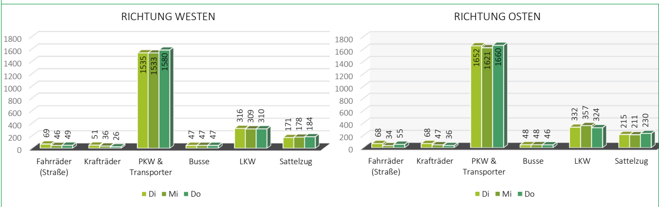
Abbildung 6: Querschnittsbelastung im westlichen Abschnitt - nachher: 04.-06.06.2019
