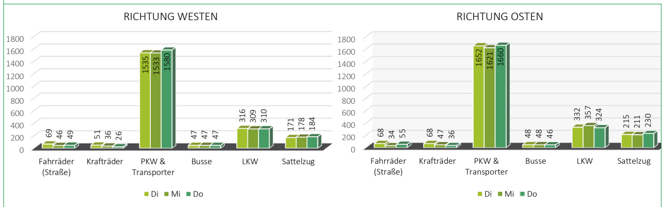
Abbildung 8: Querschnittsbelastung im östlichen Abschnitt - nachher: 4.-6.6.2019
