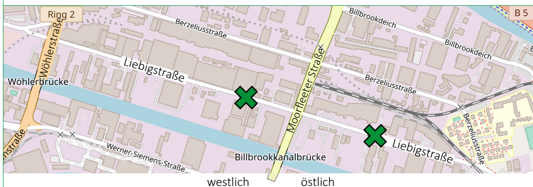
Abbildung 3: Standorte der Verkehrserhebungskameras im westlichen (links) und östlichen Abschnitt der Liebigstraße (Kartengrundlage: OpenStreetMap, Darstellung ohne Maßstab)
